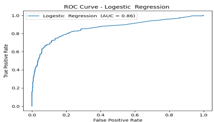
رگرسیون لجستیک
